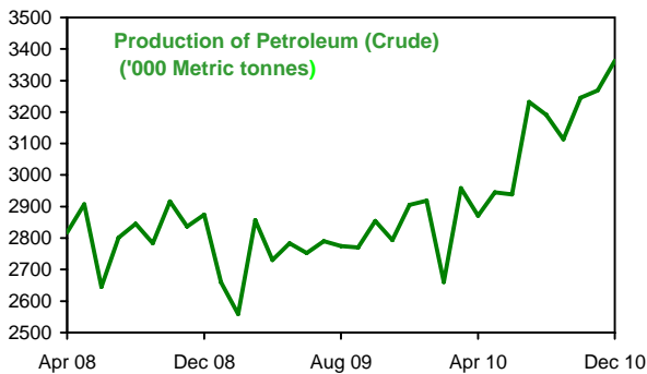
पेट्रोलियम का उत्पादन कच्चा '000मी टन
