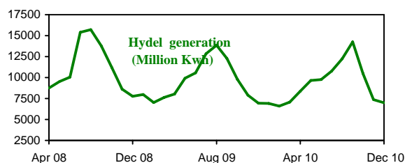
जल प्रजनित बिजली (दस लाख किलोवाटघंटे)
